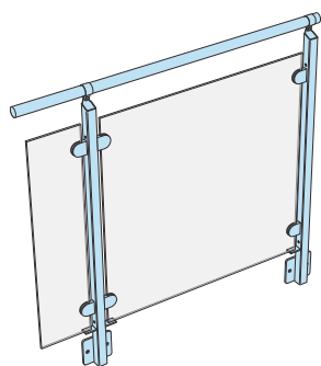
Fylling av glass.
