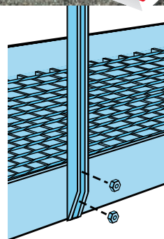
Rekkverksstenderne boltes fast i vangen.
