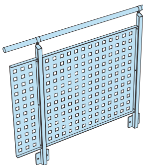
Rekkverksfylling av perforerte plater.
