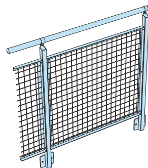
Rekkverksfylling av krenelert nett.
