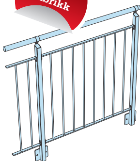
Rekkverksfylling av rundstål med maks Åpning på 100 mm.
