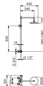
Dusjbatteri med termostat, tak- og hånddusj 150 c/c
