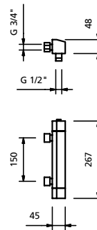
Dusjbatteri med termostat 150 c/c
