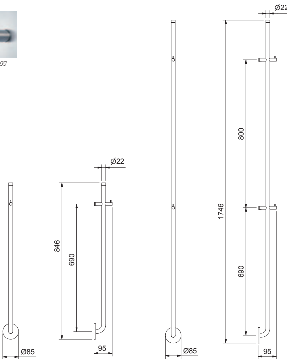
Lav modell for innebygd strøm.
