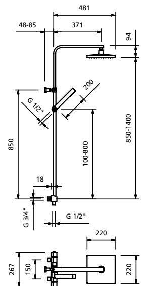
Dusjbatteri med termostat, tak- og håndduj 150 c/c
