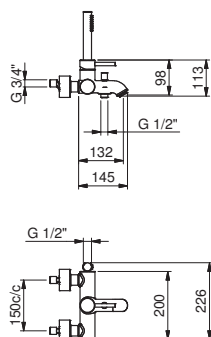
Badekarbatteri med termostat 150 c/c
