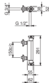
Dusjbatteri med termostat 150 c/c
