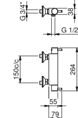
Dusjbatteri med termostat 150 c/c
