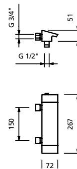
Dusjbatteri med termostat 150 c/c
