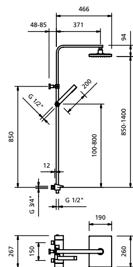
Dusjbatteri med termostat, tak- og hånddusj 150 c/c
