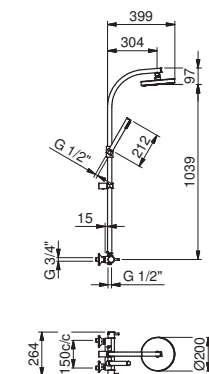
Dusjbatteri med termostat, tak- og hånddusj 150 c/c
